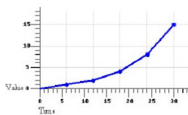
Fig. 2: linear function
